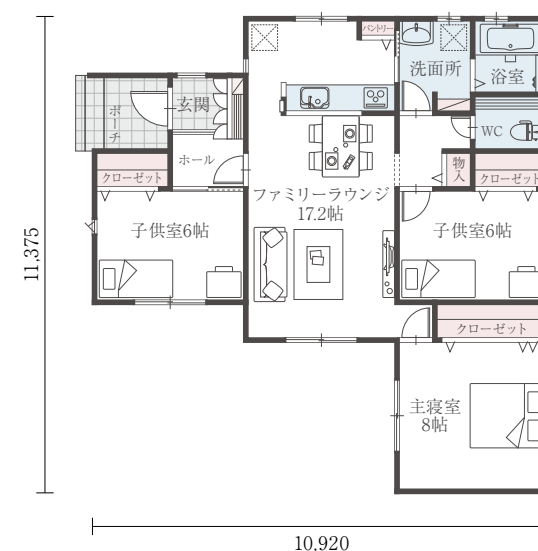
H24-EW 018/26 間口:10.92m 奥行:11.37m 床面積 26.00坪
