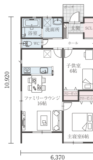
H24-N 005/19 間口:6.37m 奥行:10.92m 床面積 19.75坪
