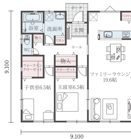
H24-N 014/24 間口:9.10m 奥行:9.10m 床面積 24.50坪
