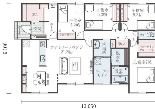
H24-EW 022/35 間口:13.65m 床面積 奥行:9.10m 35.00坪
