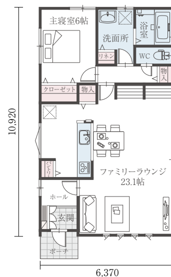
H24-S 005/20 間口:6.37m 奥行:10.92m 床面積 20.875坪
