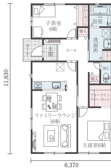
H24-EW 008/22 間口:6.37m 奥行:11.83m 床面積 22.25坪
