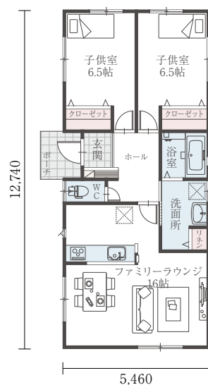
H24-EW 004/20 間口:5.46m 奥行:12.74m 床面積 20.75坪
