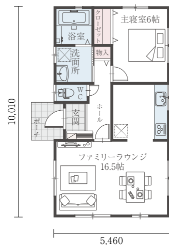
H24-EW 001/16 間口:5.46m 奥行:10.01m 床面積 16.25坪
