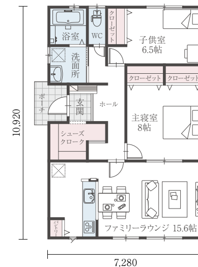
H24-EW 012/23 間口:7.28m 奥行:10.92m 床面積 23.50坪
