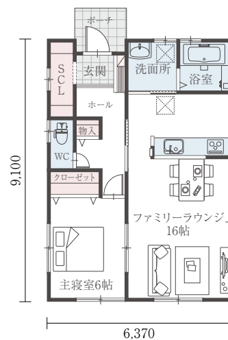
H24-N 002/17 間口:6.37m 奥行:9.10m 床面積 17.25坪
