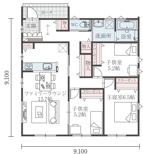
H24-N 016/25 間口:9.10m 奥行:9.10m 床面積 25.00坪
