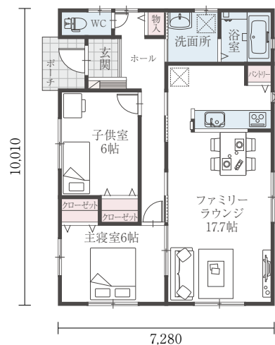
H24-EW 007/21 間口:7.28m 奥行:10.01m 床面積 21.50坪
