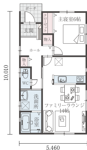
H24-N 001/16 間口:5.46m 奥行:10.01m 床面積 16.00坪
