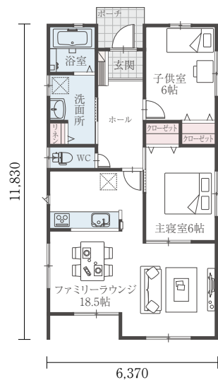
H24-N 007/21 間口:6.37m 奥行:11.83m 床面積 21.50坪
