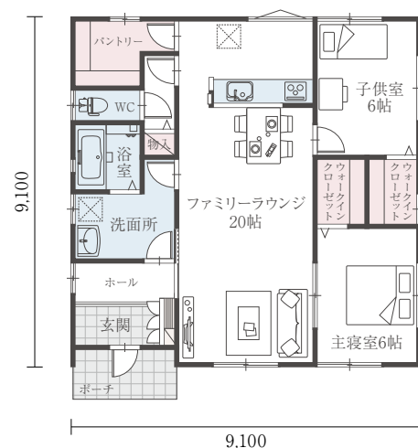
H24-S 014/24 間口:9.10m 奥行:9.10m 床面積 24.63坪
