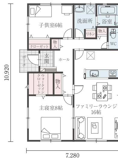
H24-EW 011/23 間口:7.28m 奥行:10.92m 床面積 23.50坪
