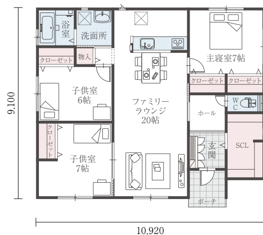
H24-S 023/28 間口:10.92m 奥行:9.1m 床面積 28.75坪
