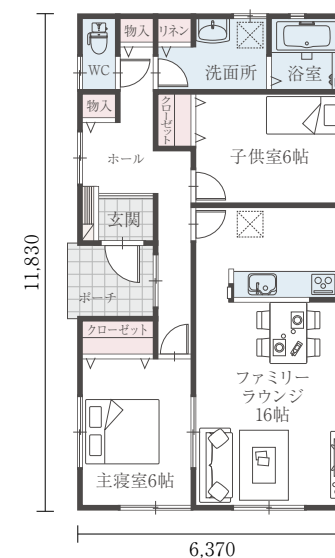
H24-EW 006/21 間口:6.37m 奥行:11.83m 床面積 21.75坪
