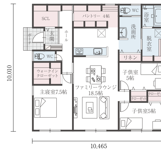
H24-EW 021/31 間口:10.46m 床面積 奥行:10.01m 31.13坪
