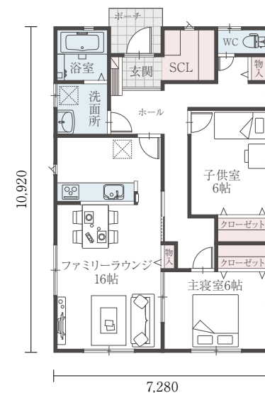
H24-N 012/23 間口:7.28m 奥行:10.92m 床面積 23.50坪
