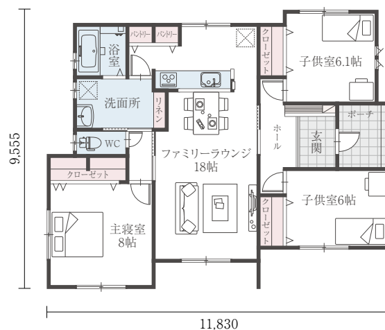
H24-EW 020/27 間口:11.83m 床面積 奥行:9.55m 27.19坪
