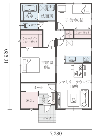
H24-S 013/23 間口:7.28m 奥行:10.92m 床面積 23.75坪
