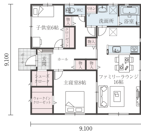
H24-EW 016/24 間口:9.10m 奥行:9.10m 床面積 24.75坪
