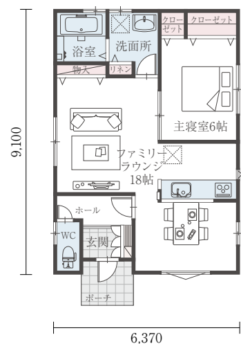
H24-S 001/17 間口:6.37m 奥行:9.10m 床面積 17.25坪
